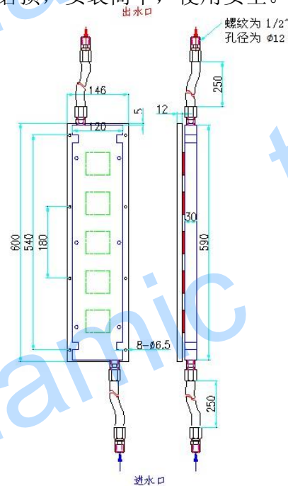
50W 热电半导体发电机结构图
